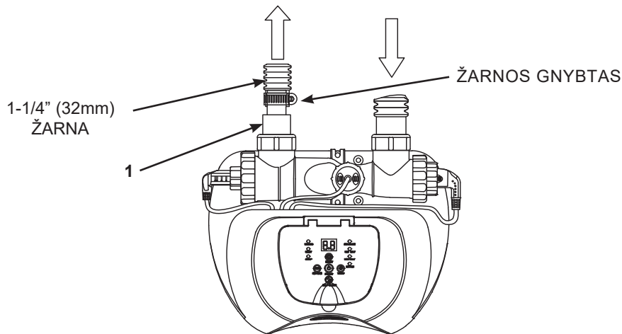
SŪRAUS VANDENS SISTEMA SU E.C.O. (ELEKTROKATALIZINE OKSIDACIJA)
